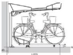
■断面図(下段) 前・後入れタイプ JCR-SFB-1型
