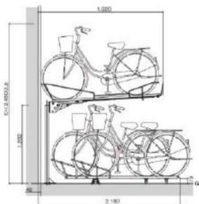
■断面図(下段) 前入れタイプ JCR-SF-1型
