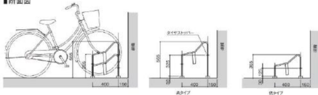
■断面図
